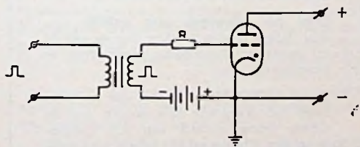
Fig. 1. Thyratron met transformator in het stuur elektrode-circuit. Via deze transformator kan de ontsteek-impuls aan deze elektrode worden toegevoerd.
