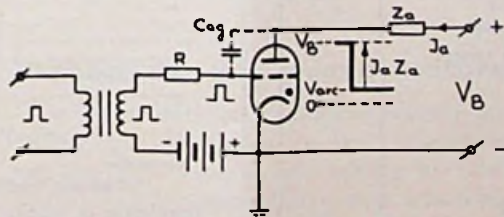
Fig. 2. Dezelfde schakeling als in fig. 1, waarin echter het spanningsverloop is aangegeven aan de anode in het geval van het ontsteken van het thyratron. Via de anode-rooster capaciteit wordt de spanningsstoot aan de anode teruggevoerd naar de stuur elektrode.
