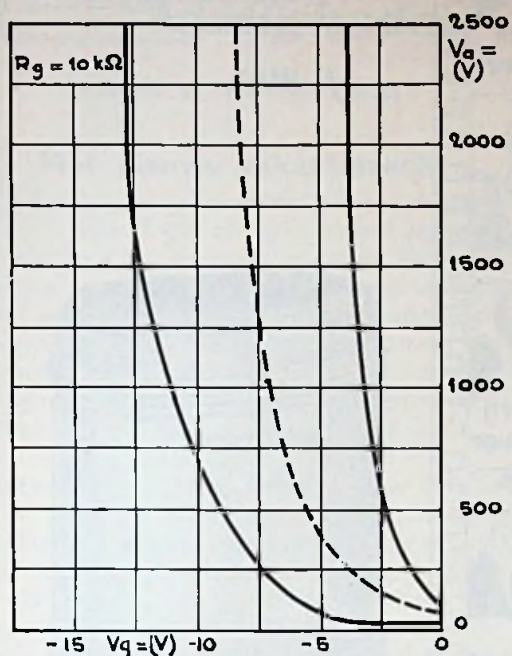
Fig. 3. Ontsteekarakteristiek van het Philips thyatron PL 5557.
